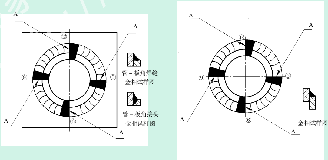
图 A-8 管板角接头和管材角焊缝试件金相试样(宏观)的截取位置
