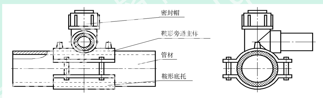
(d) 电熔连接焊鞍形试件(旁通式) 代号 A
