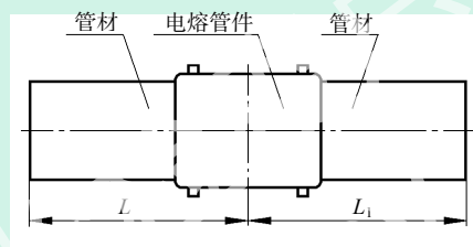
(c) 电熔连接焊承插试件 代号 C
