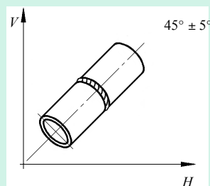
(d) 45° 固定试件 代号 6G、6GX(向下焊)
