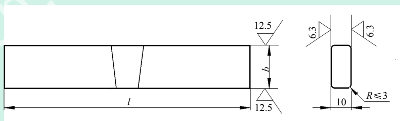
(c) 横向侧弯试样
