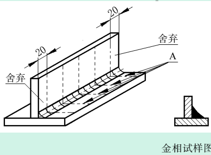
图 A-9 板材角焊缝试件金相试样(宏观)截取位置
