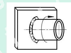
(c) 水平转动试件 代号 2FR (转动)
