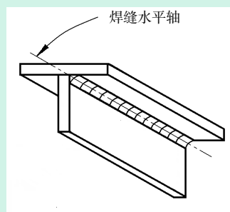
(d) 仰焊试件 代号 4F
