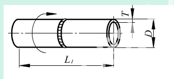
(a) 水平转动试件 代号 1G(转动)
