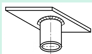
(d) 垂直固定仰焊试件 代号 4F
