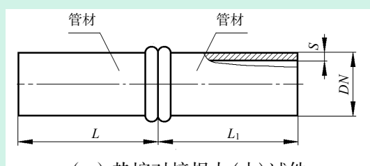
(a) 热熔对接焊大(小)试件 代号 D 或者 d
