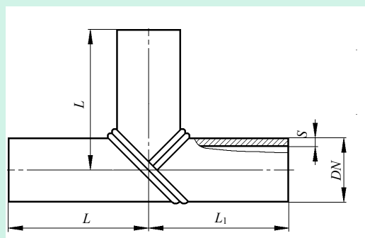
(b) 热熔对接焊三通试件 代号 S
