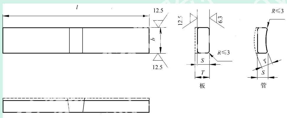
(b) 板状和管状试件的背弯试样
