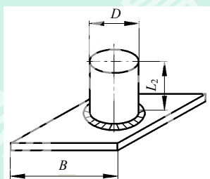
(a) 平焊试件 代号 1S
