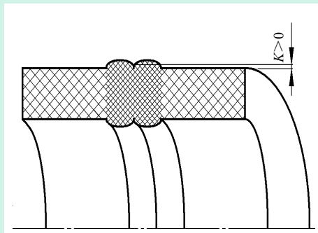
图 B-2 对接焊卷边示意图
