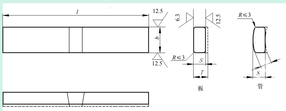
(a) 板状和管状试件的面弯试样
