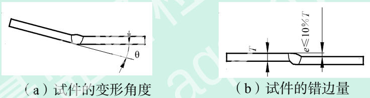
图 A-4 板材试件的变形角度和错边量
