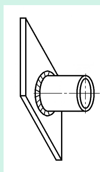
(d) 水平固定试件 代号 5FG
