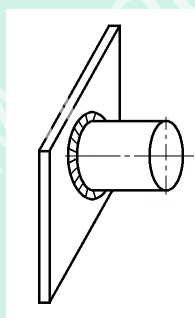
(b) 横焊试件 代号 2S
