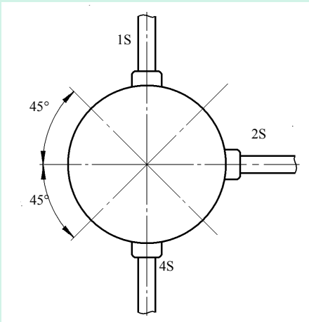
图 A-3 螺柱焊焊件焊接位置范围
