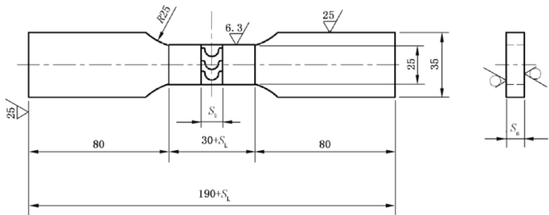
图 10 拉伸试样图
