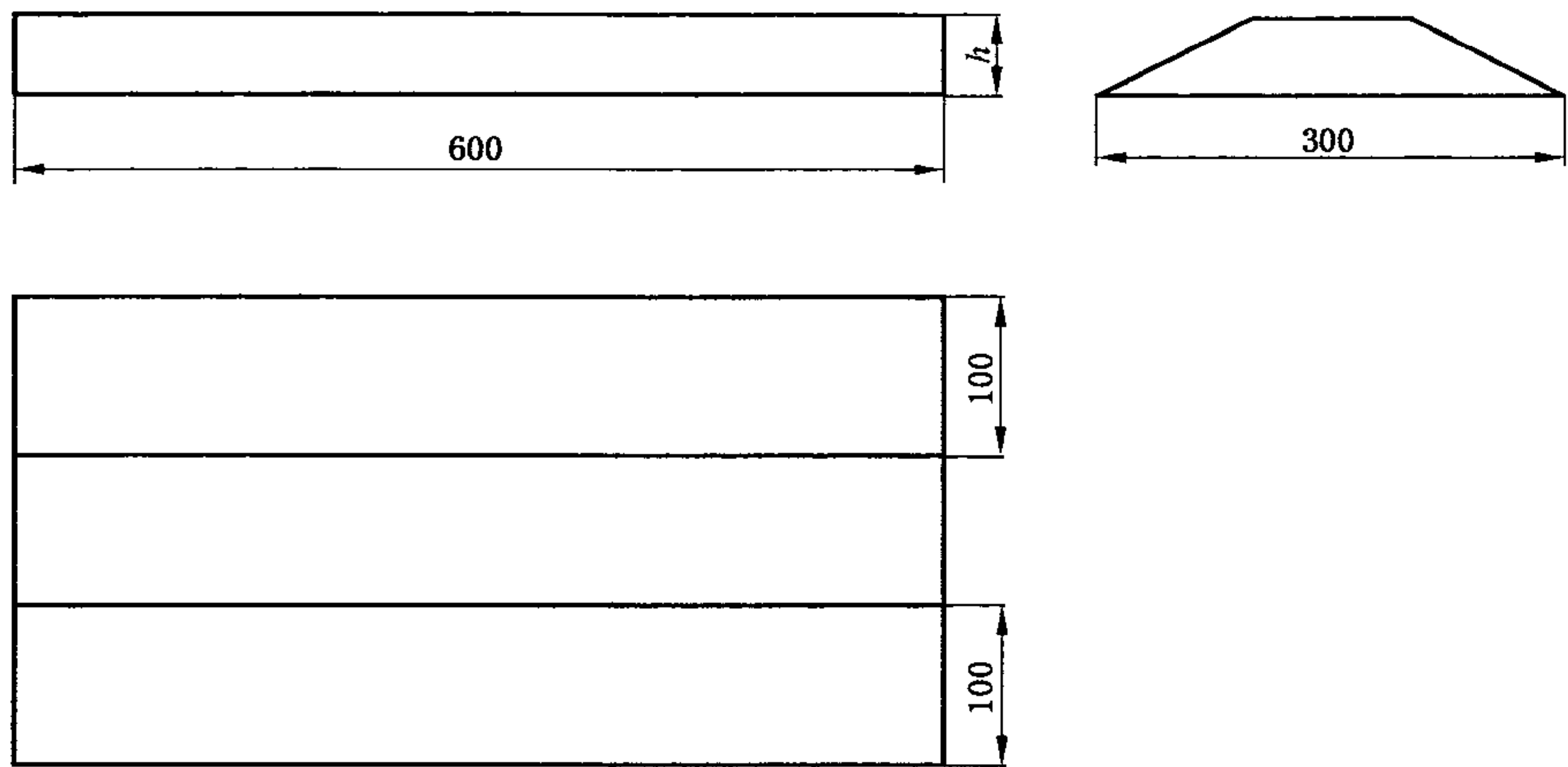
图 4 障碍块尺寸
